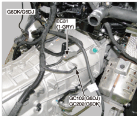
53. 变速器右侧
