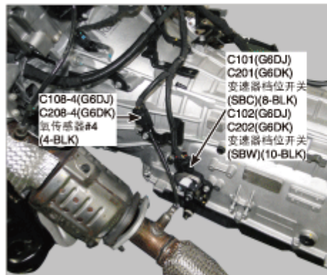
52. 变速器左侧
