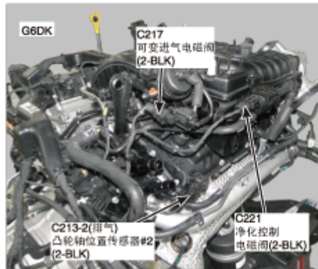
49. 发动机后右
