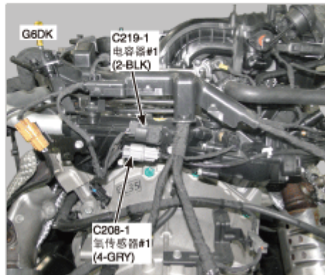
51. 发动机后部
