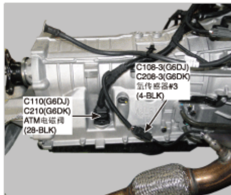
54. 变速器右侧
